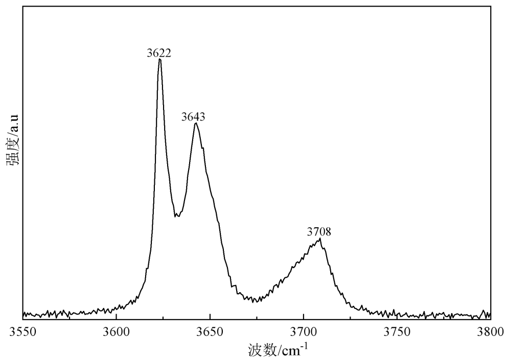
图 B. 3 迪开石高频区的拉曼光谱
