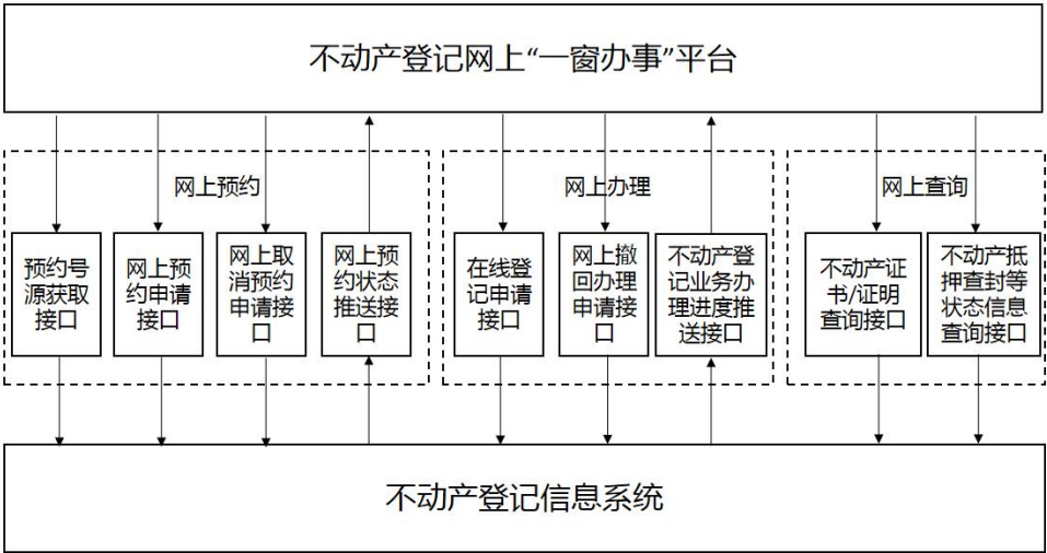
图1 接口构成图
