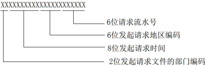
图 1 查询请求单号
