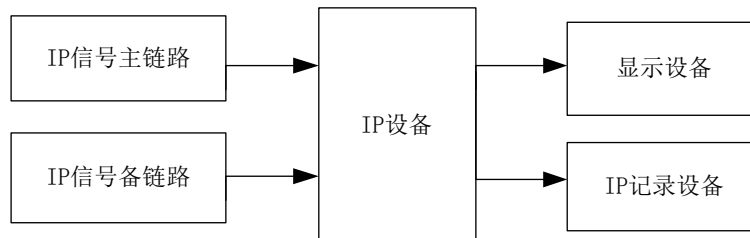
图26 冗余备份 IP 流倒换测量框图
